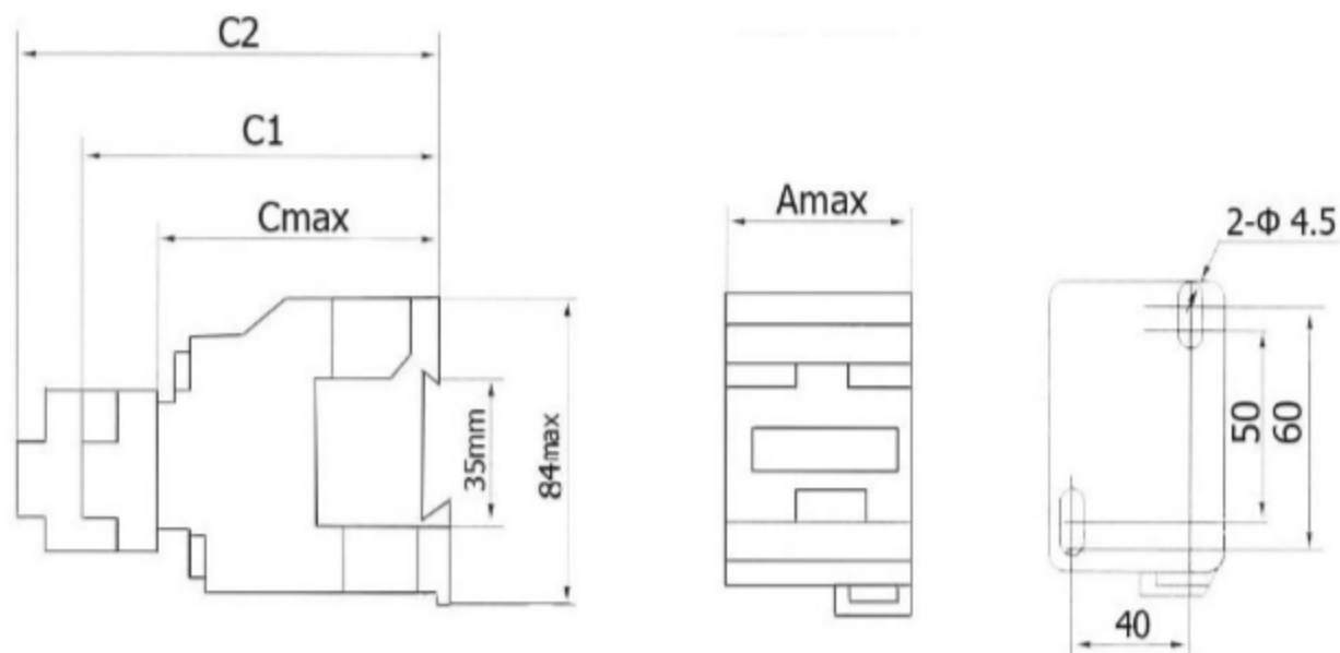
Рисунок 3 - Габаритные и присоединительные размеры пускателей 16-40А
