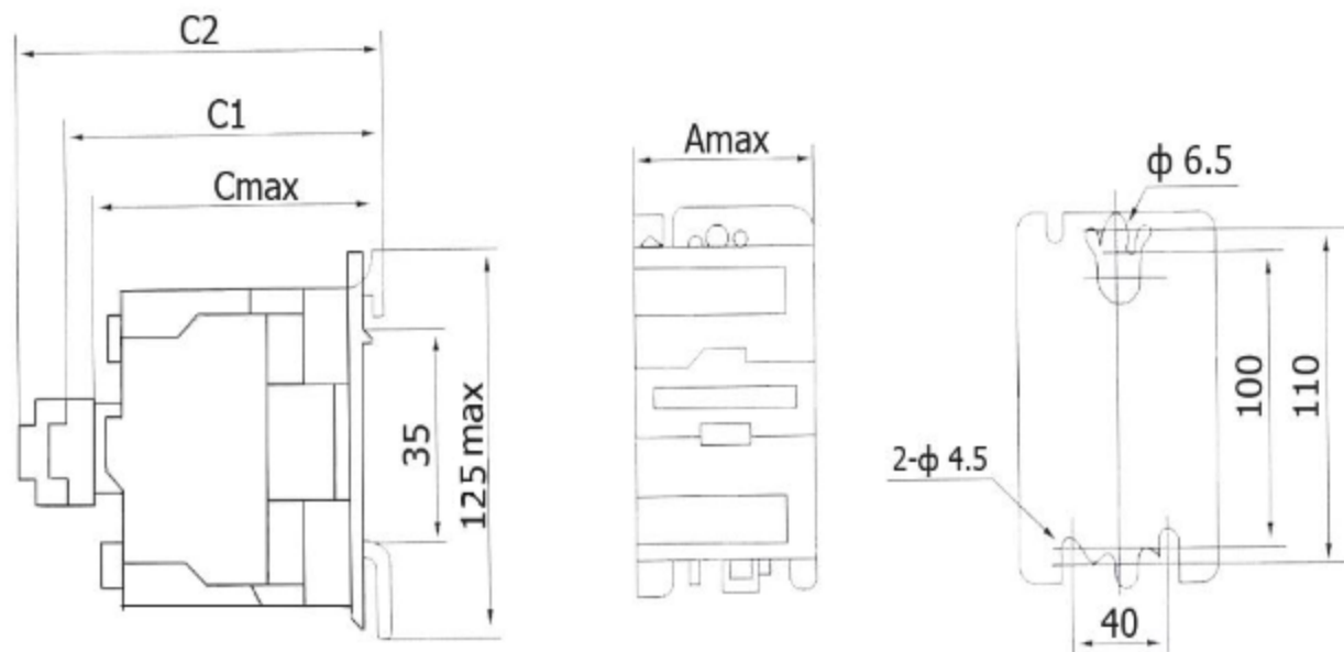
Рисунок 4 - Габаритные и присоединительные размеры пускателей 40-95А
