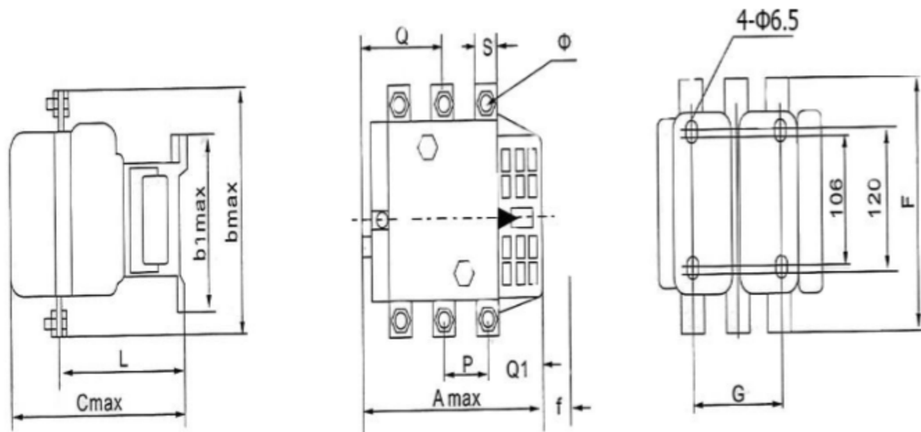
Рисунок 5 - Габаритные и присоединительные размеры пускателей 160-250А
